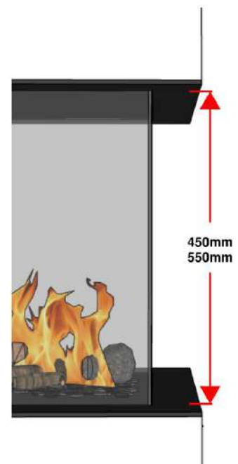
Tussenmaat
